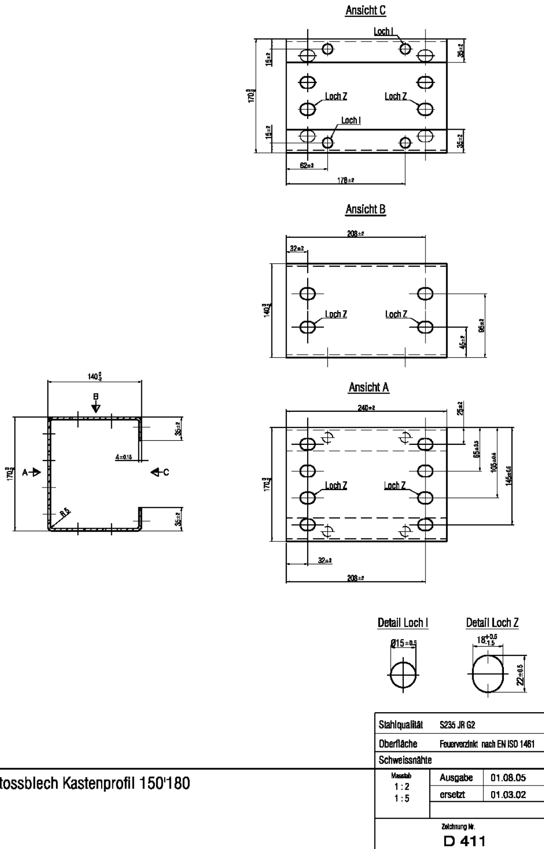
Abb. 2.10 Stossblech Kastenprofil 150*180.
