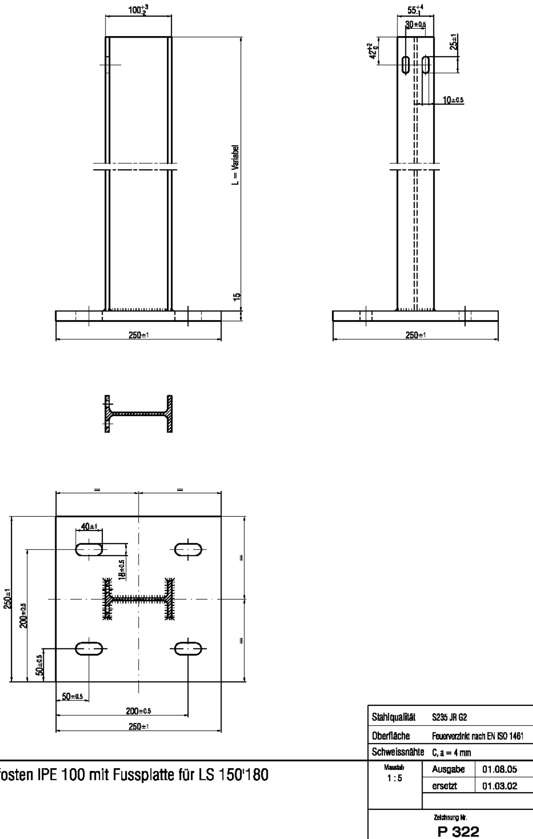
Abb. 2.7 Pfosten IPE mit Fussplatte.
