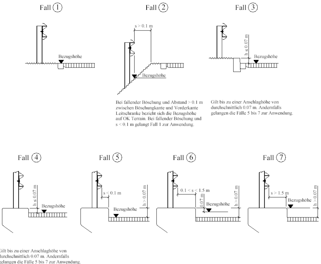
Abb. 6.10 Einbauhöhen.
